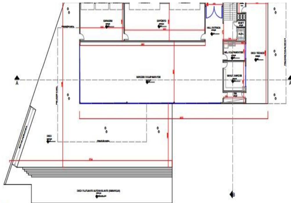
PLANTA BAIXA PAV. TÉRREO S.C. 1102
